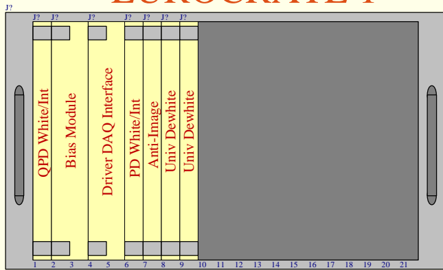
EUROCRATE
