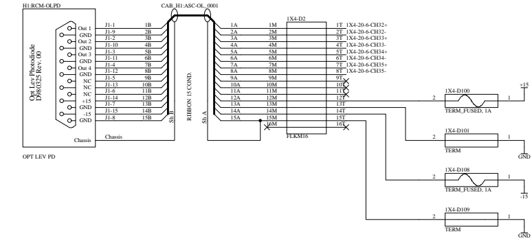
LHO 4K BS Opt Lever PD
