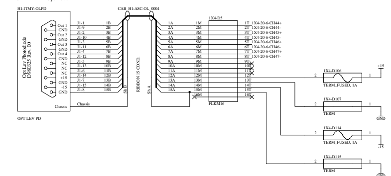
LHO 4K ITMY Opt Lever PD
