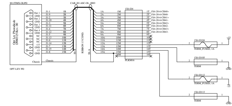
LHO 4K ITMX Opt Lever PD
