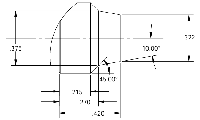
DETAIL DE SCALE 4 : 1
