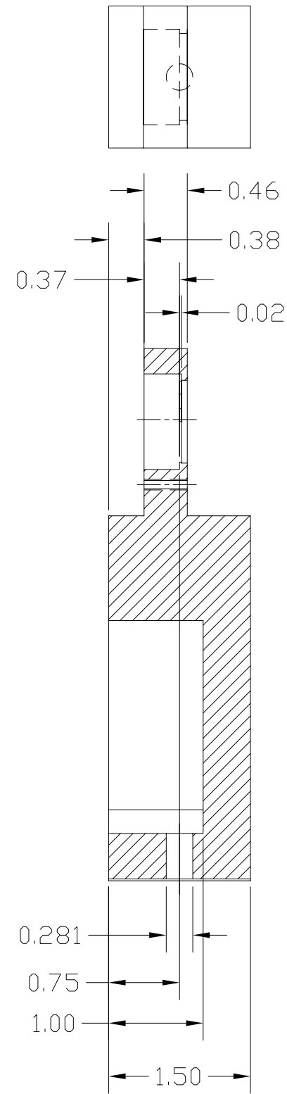
SECTION A-A
