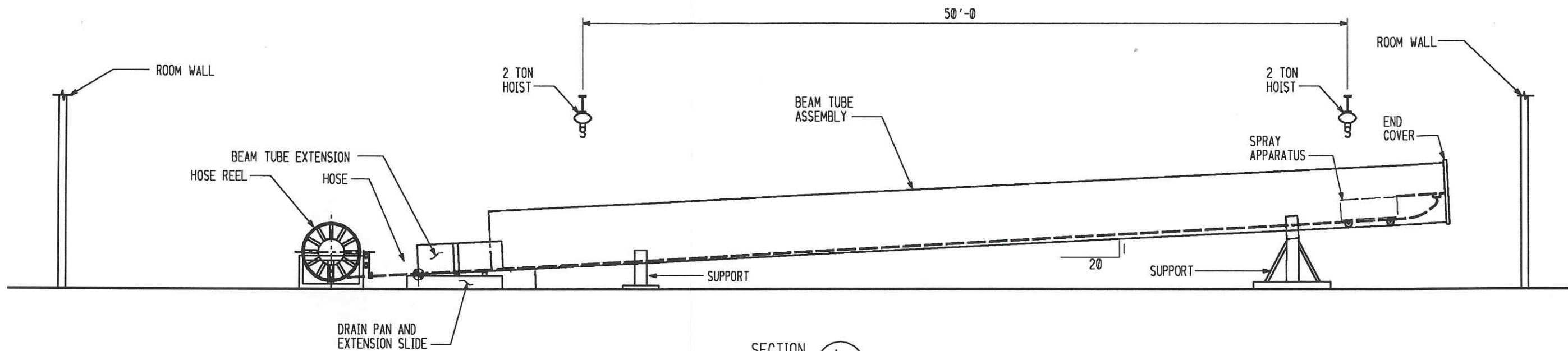
SECTION A SHT 1
