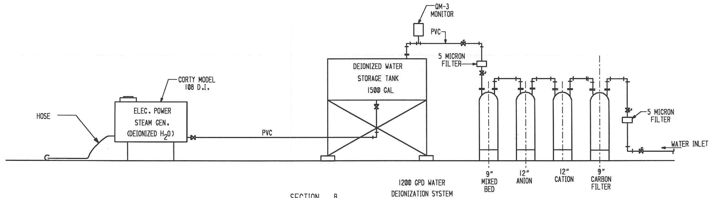
SECTION B SHT 1
