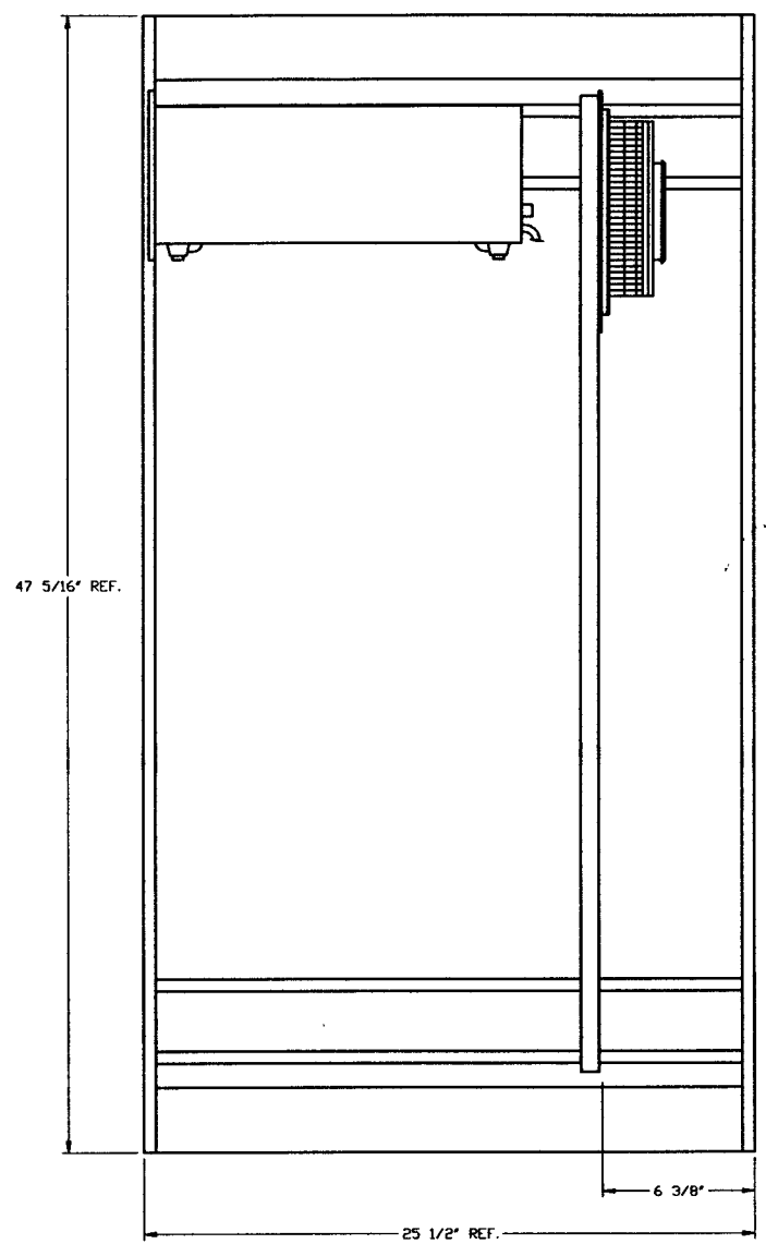
SECTION A-A
