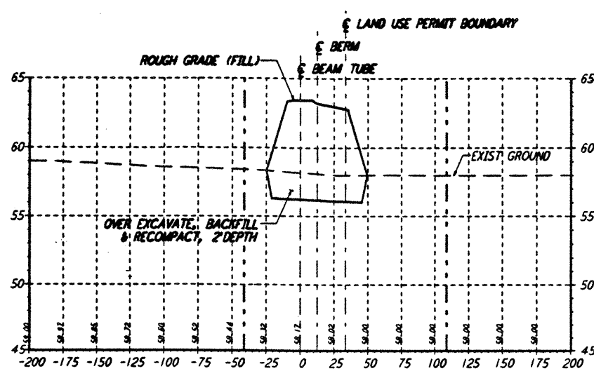
STA 6+00.00
