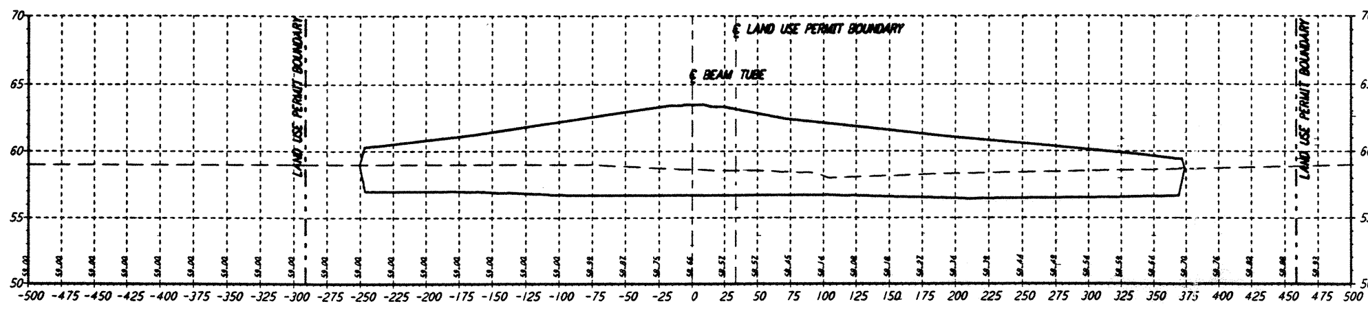
STA 4+00.00
