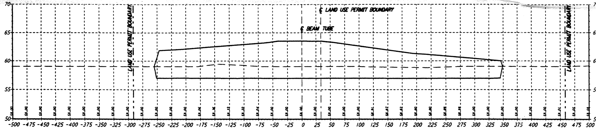
STA 2+00.00
