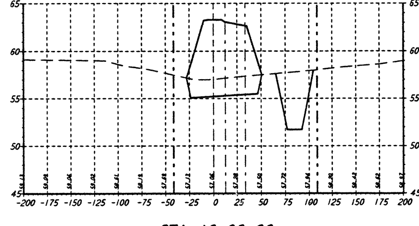
STA 10+00.00
