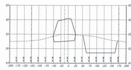
STA 70+00.00
