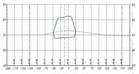
STA 50+00.00
