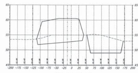
STA 66+00.00
