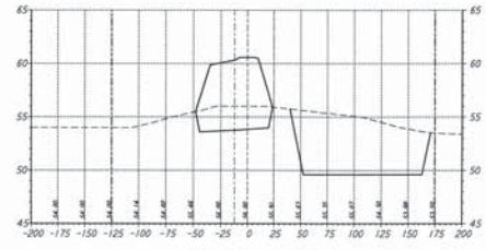
STA 64+00.00
