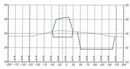
STA 62+00.00
