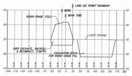
STA 56+00.00
