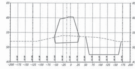
STA 72+00.00
