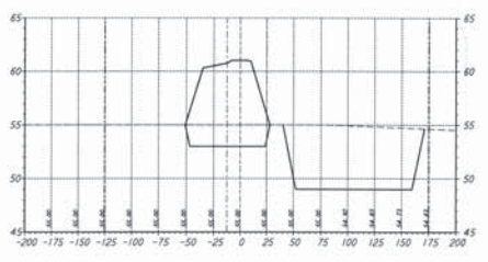
STA 52+00.00
