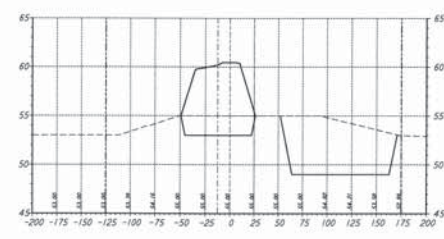
STA 68+00.00
