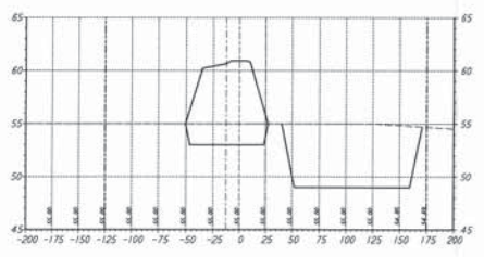
STA 54+00.00
