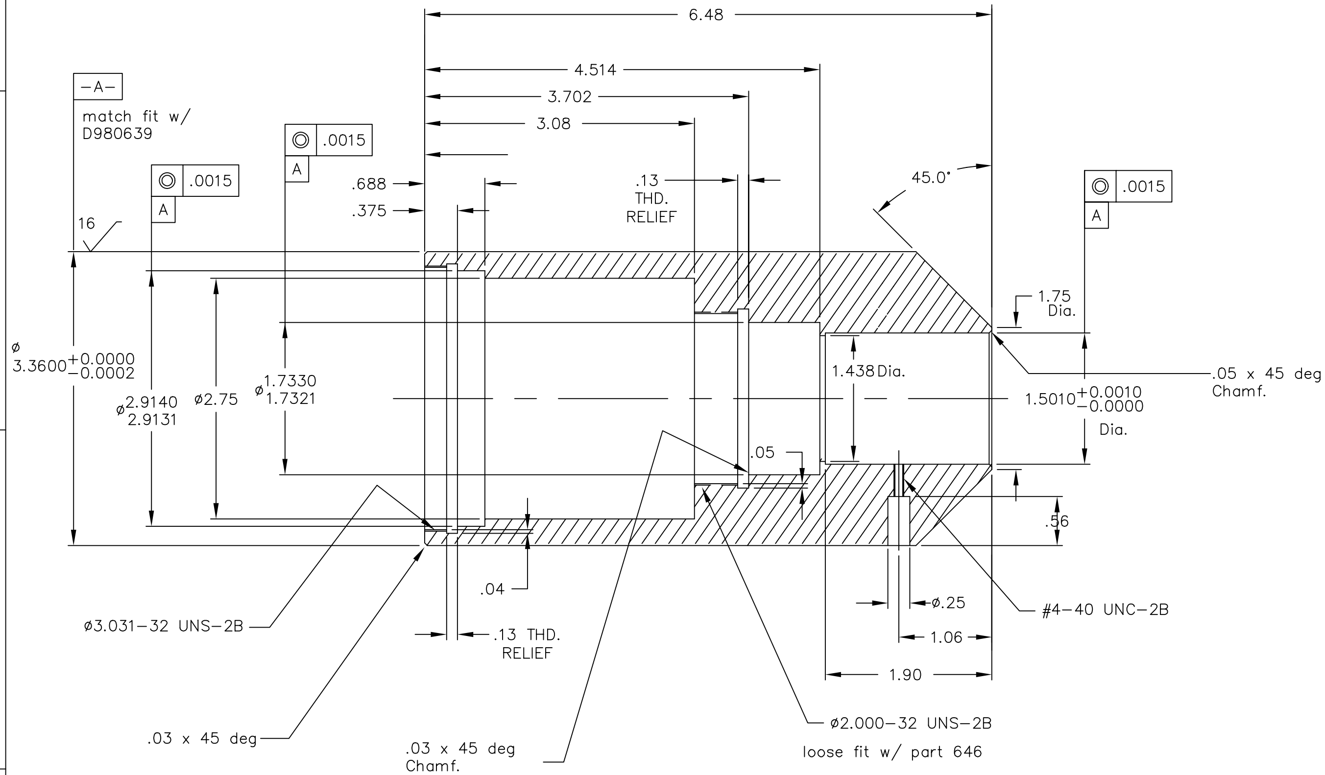
SECTION A-A
