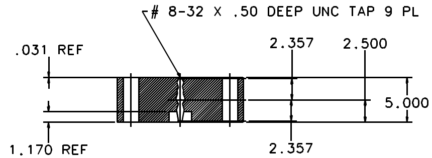
VIEW A-A
