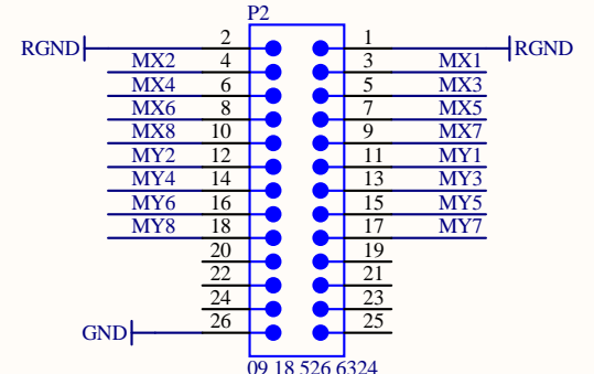
DB25/male
