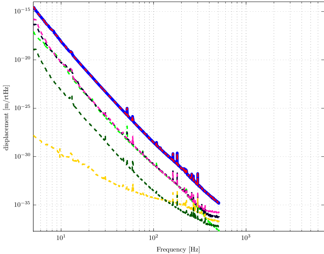
ETMX NoiseBudget
