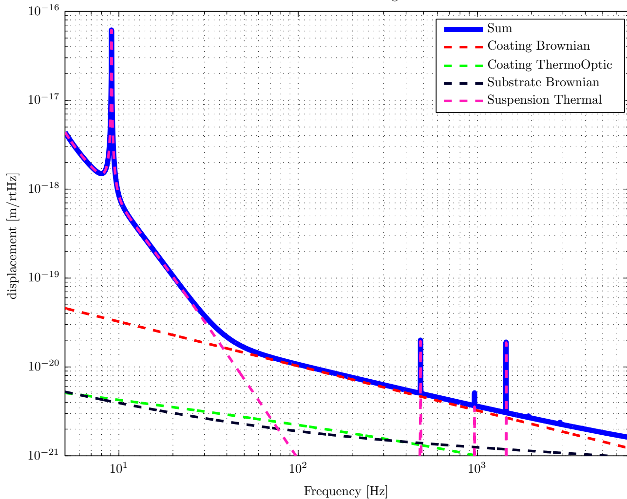
Thermal NoiseBudget
